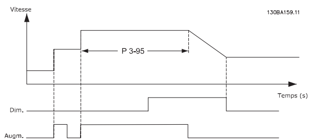
Illustration 3.23 Cas n° 2 de retard de rampe
