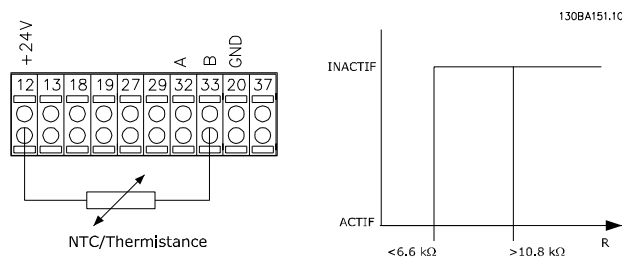
Illustration 3.15 Connexion de la thermistance
