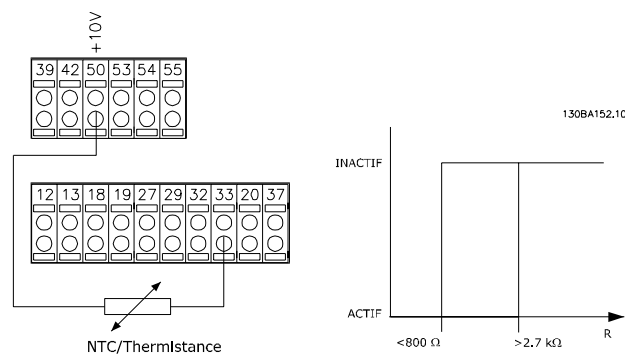
Illustration 3.12 Connexion de la thermistance PTC - entrée digitale
