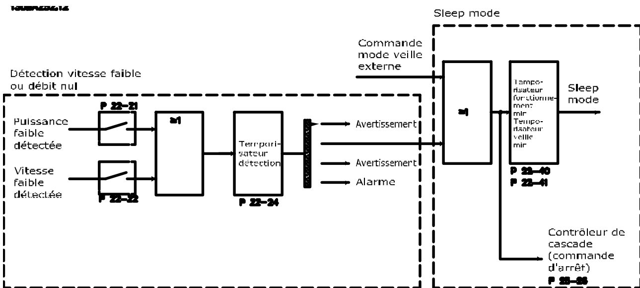
Illustration 3.50 Détection d'absence de débit
