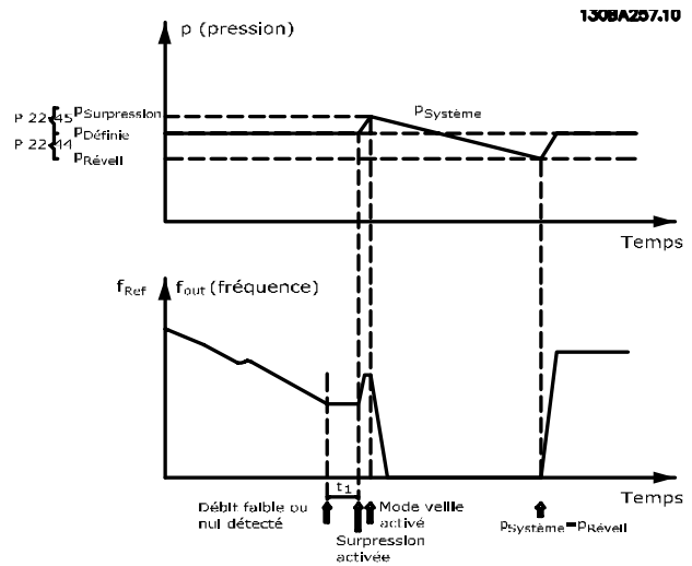
Illustration 3.52 Système de suralimentation
