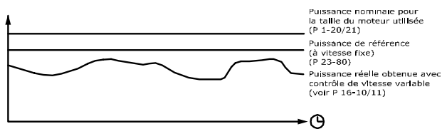
Illustration 3.65 Commande de vitesse variable
