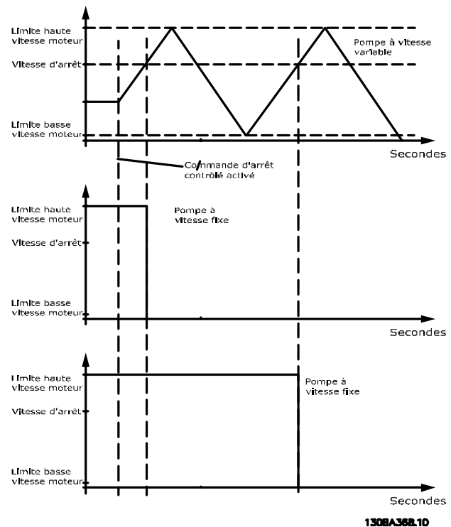
Illustration 3.80 Vitesse d'arrêt
