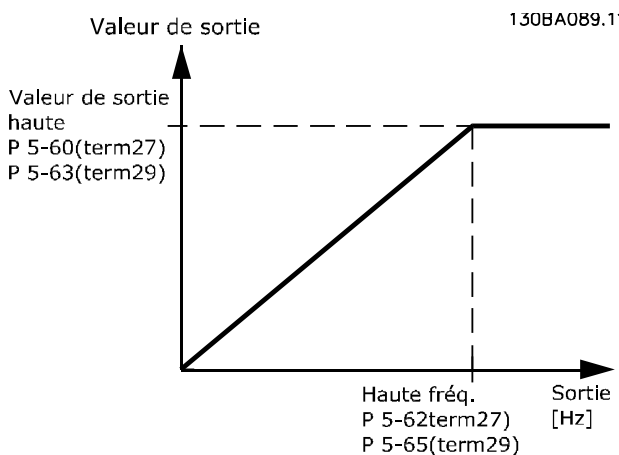
Illustration 3.28 Sortie impulsions
