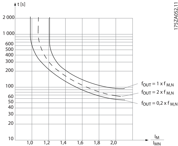
Illustration 3.10 Protection thermique du moteur
