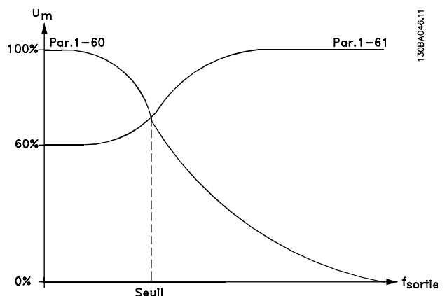
Illustration 3.9 Compensation de la charge à faible vitesse
