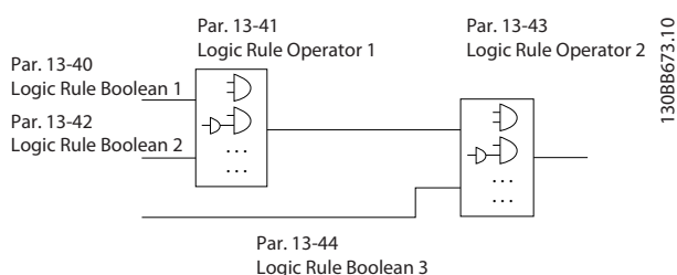
Illustration 3.36 Règles logiques
