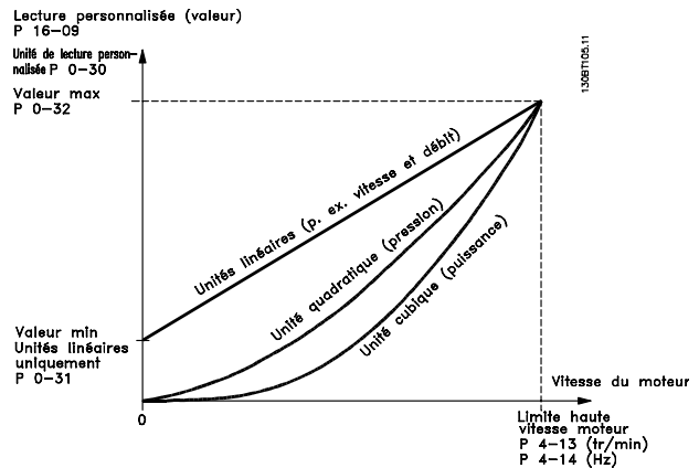
Illustration 3.3 Lect.paramétr.
