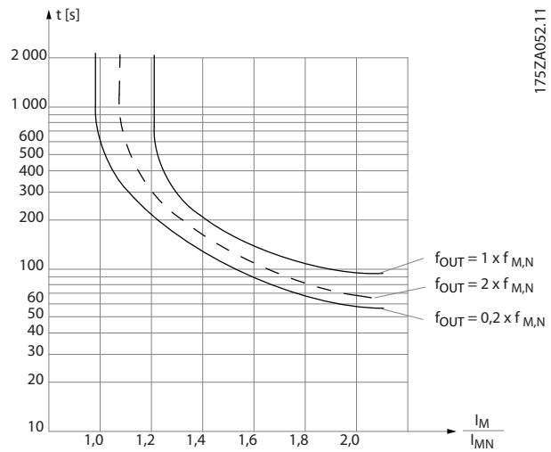
Illustration 3.14 Profil ETR
