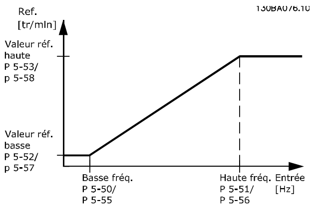
Illustration 3.27 Entrée impulsions
