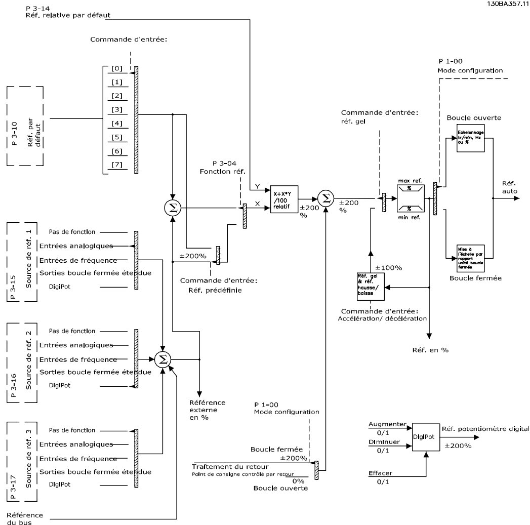
Illustration 3.17 Exemple de fonctionnement en boucle ouverte ou fermée
