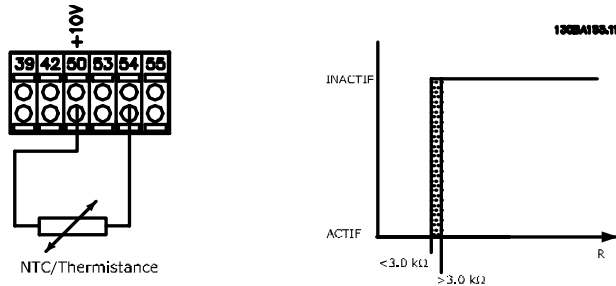
Illustration 3.13 Connexion de la thermistance PTC - entrée analogique
