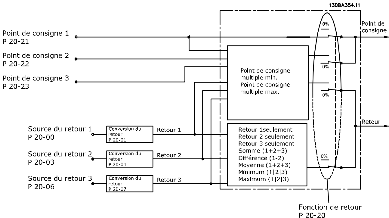
Illustration 3.47 Signal de retour
