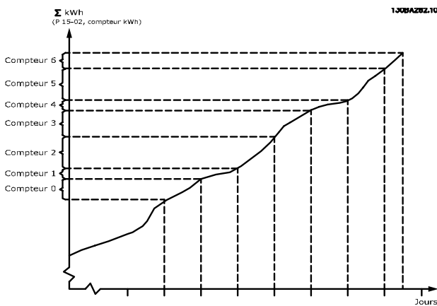
Illustration 3.62 Graphique du journal énergétique
