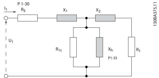
Illustration 3.4 Schéma moteur équivalent pour un moteur asynchrone
