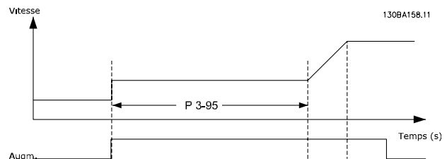
Illustration 3.22 Cas n° 1 de retard de rampe
