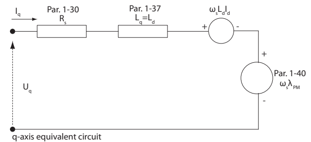
Illustration 3.5 Schéma de câblage moteur équivalent pour un moteur PM non saillant
