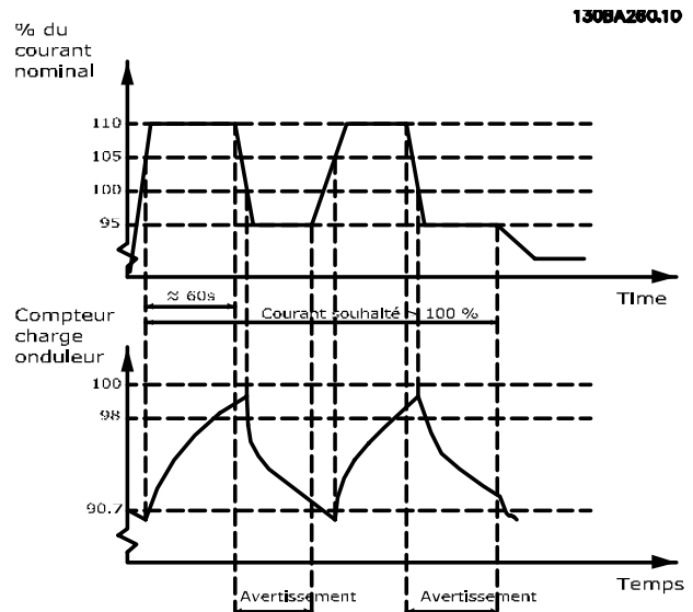
Illustration 3.43 Courant de sortie en condition de surcharge
