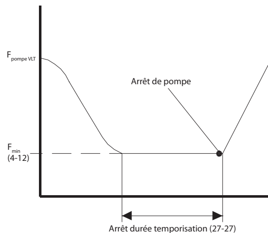
Illustration 3.75 Durée fonct. d'arrêt
