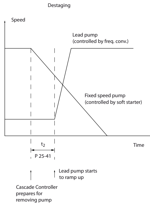
Illustration 3.77 Arrêt
