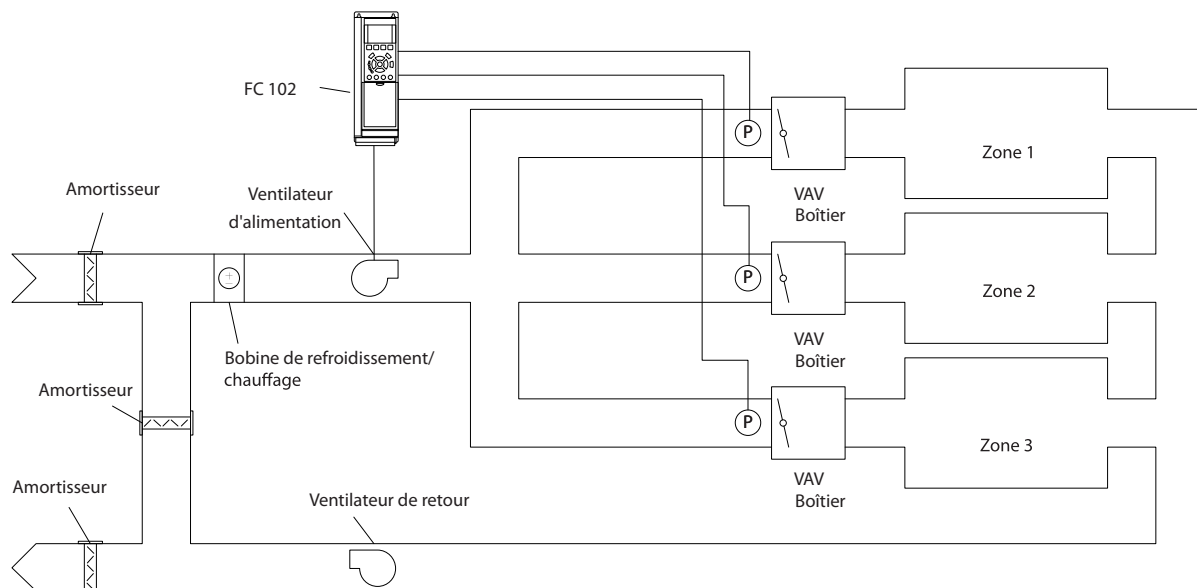
Illustration 3.48 Exemple - Multizones, une seule consigne
