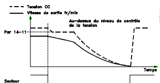
Illustration 3.40 Sauvegarde cinétique, panne secteur plus longue
