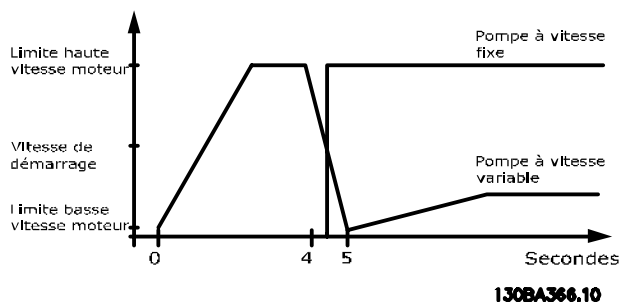
Illustration 3.78 Seuil de démarrage
