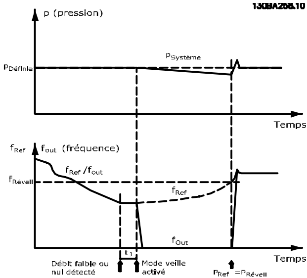
Illustration 3.54 Système de suralimentation
