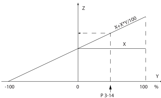
Illustration 3.19 Référence réelle
