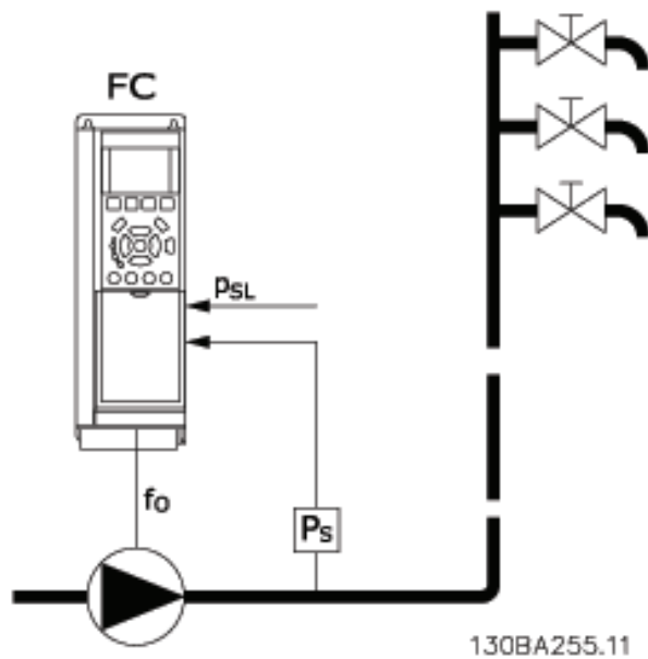
Illustration 3.51 Fonction mode veille
