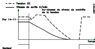
Illustration 3.38 Rampe de décélération ctrlée, défaut secteur plus long
