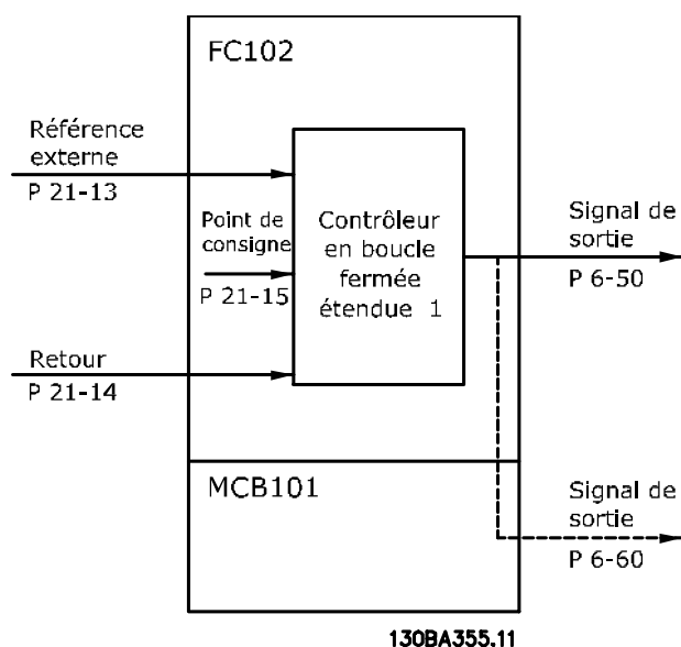
Illustration 3.49 Réf/ret PID ét. 1
