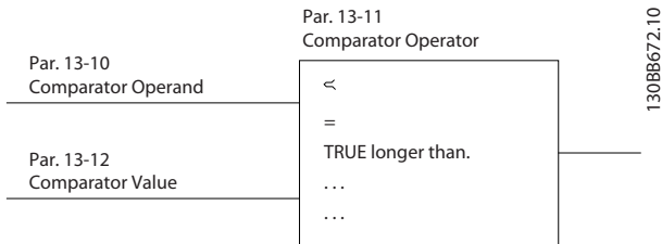
Illustration 3.35 Comparateurs
