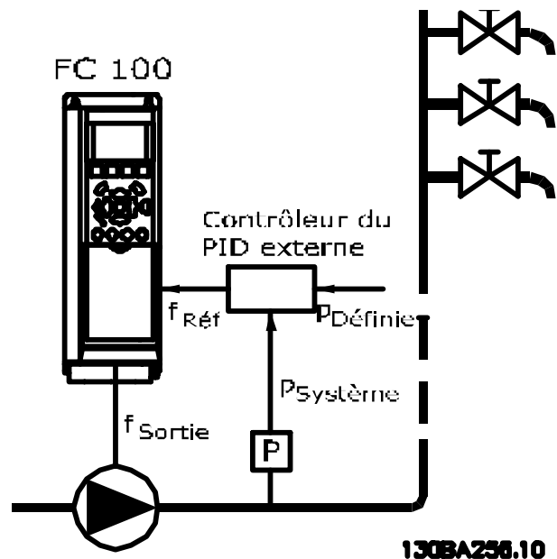
Illustration 3.53 Système de suralimentation
