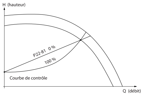
Illustration 3.57 Approx. courbe linéaire-quadratique
