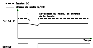
Illustration 3.39 Sauvegarde cinétique, brève panne de secteur
