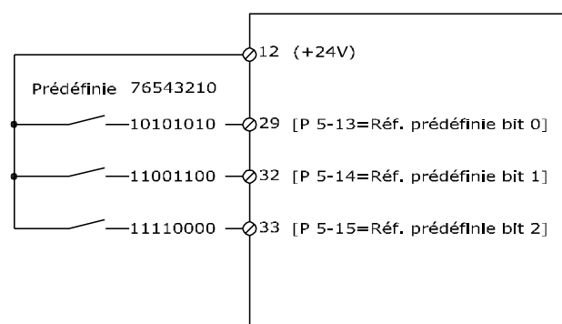
Illustration 3.16 Schéma de références prédéfinies
