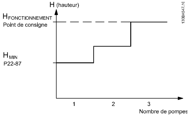
Illustration 3.56 Nombre de pompes
