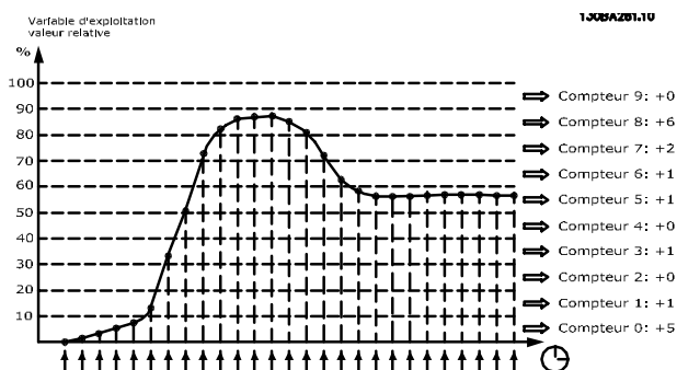
Illustration 3.64 Heure et valeurs relatives
