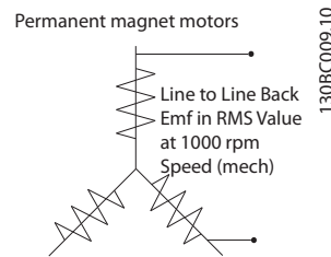
Illustration 3.7 Définitions des paramètres machine de la FCEM des moteurs PM
