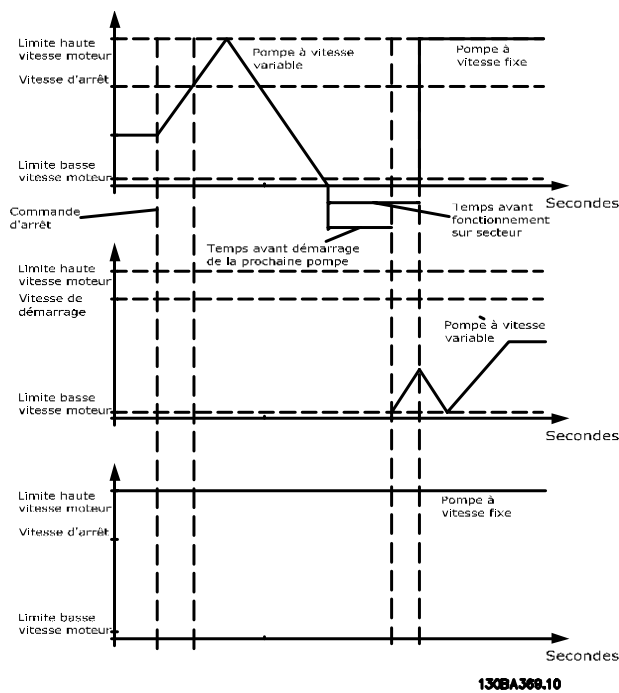
Illustration 3.81 Mode démarr. sur alternance
