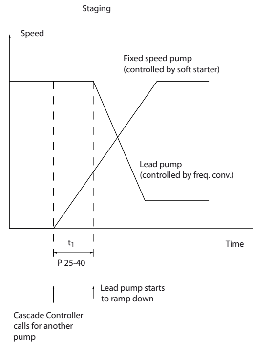
Illustration 3.76 Démarrage
