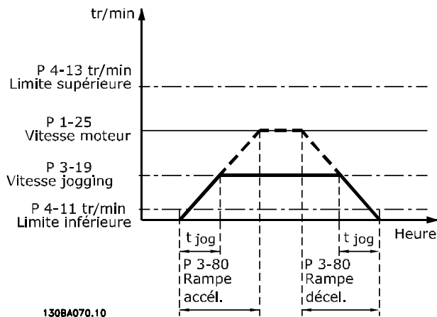
Illustration 3.21 Temps de la rampe de jogging
