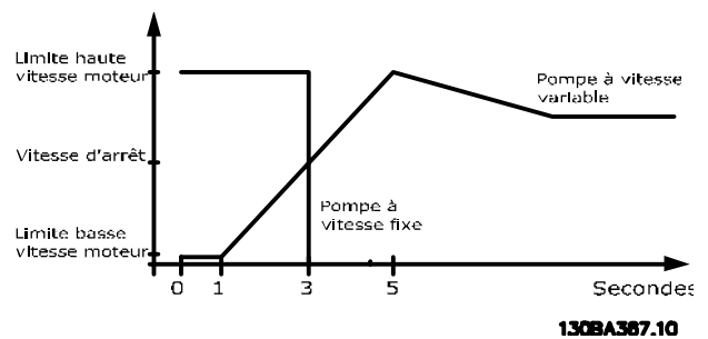
Illustration 3.79 Seuil d'arrêt
