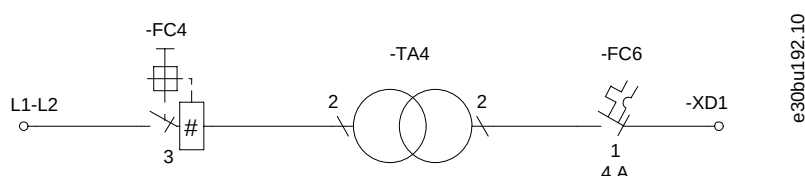
Illustration 43: Bornes de transformateur de tension auxiliaire
