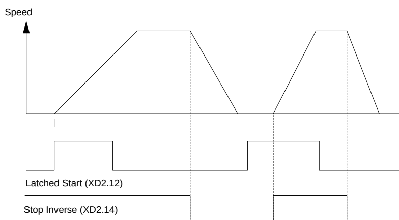
Illustration 62: Démarrage par impulsion/arrêt
