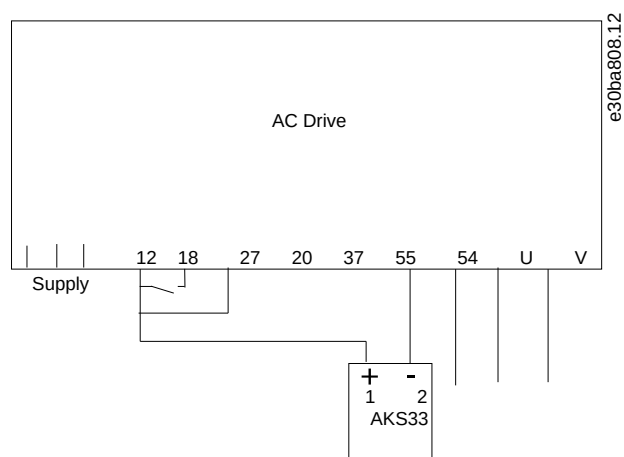
Illustration 67: Connexion du FC 103 et de l'AKS33 pour applications en boucle fermée
