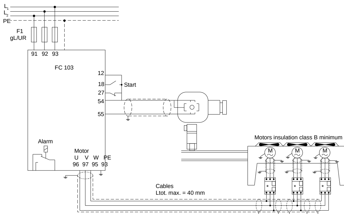
Illustration 65: Contrôle de pression en boucle fermée – Système autonome – Ventilateur ou pompe unique/ventilateurs ou pompes multiples en parallèle
