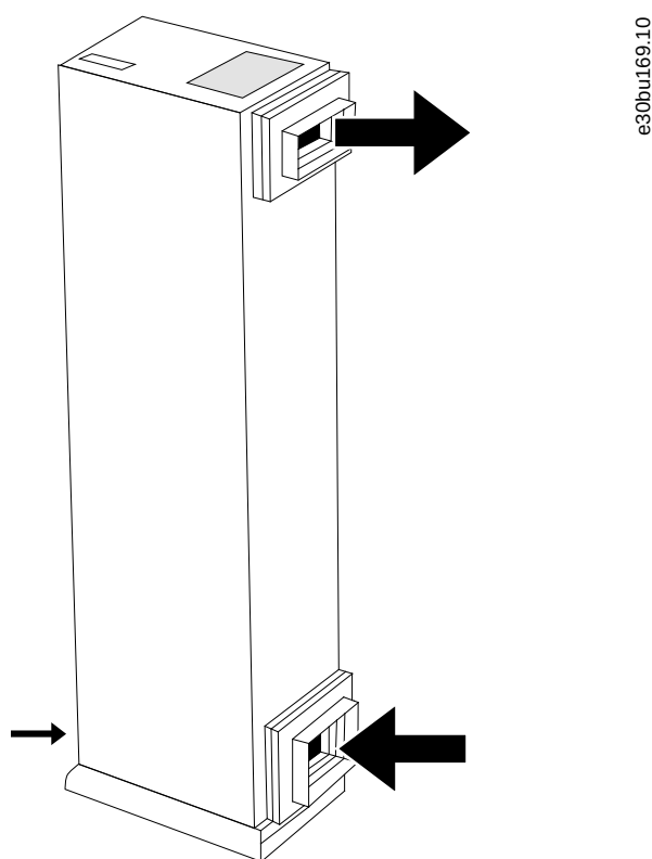
Illustration 18: Circulation d'air dans l'armoire avec option de canal de ventilation arrière (brides d'adaptation de gaine non fournies avec l'option)
