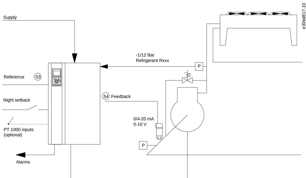
Illustration 63: Configuration standard du compresseur avec commande interne
