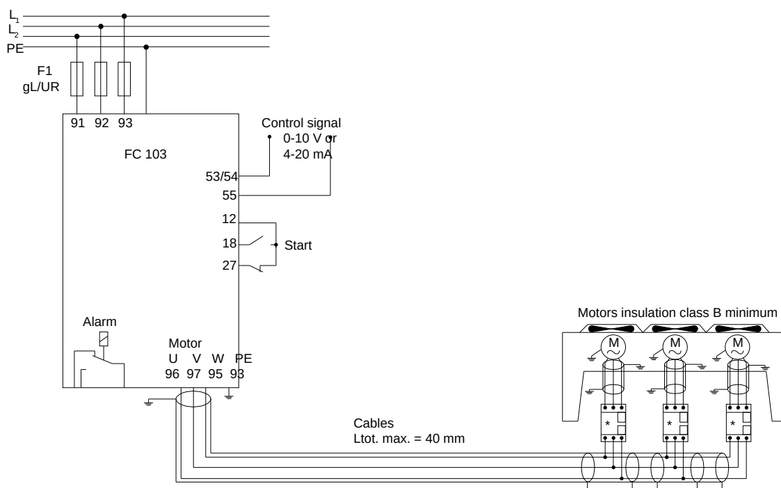
Illustration 64: Commande de vitesse utilisant la référence analogique (boucle ouverte) – Ventilateur ou pompe unique/ventilateurs ou pompes multiples en parallèle
