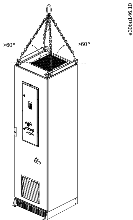
Illustration 13: Méthode de levage recommandée
