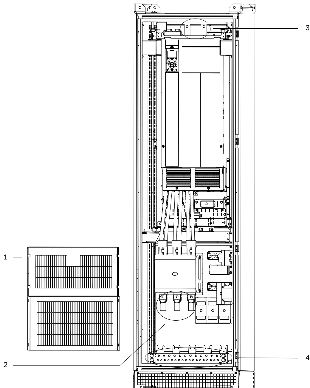
Illustration 49: Points de connexion du secteur au module variateur
